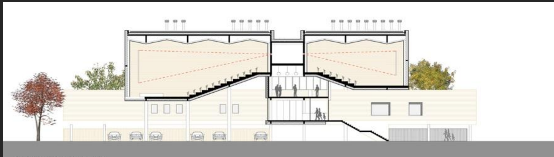
Coupe sur les salles de cinéma 1/200
