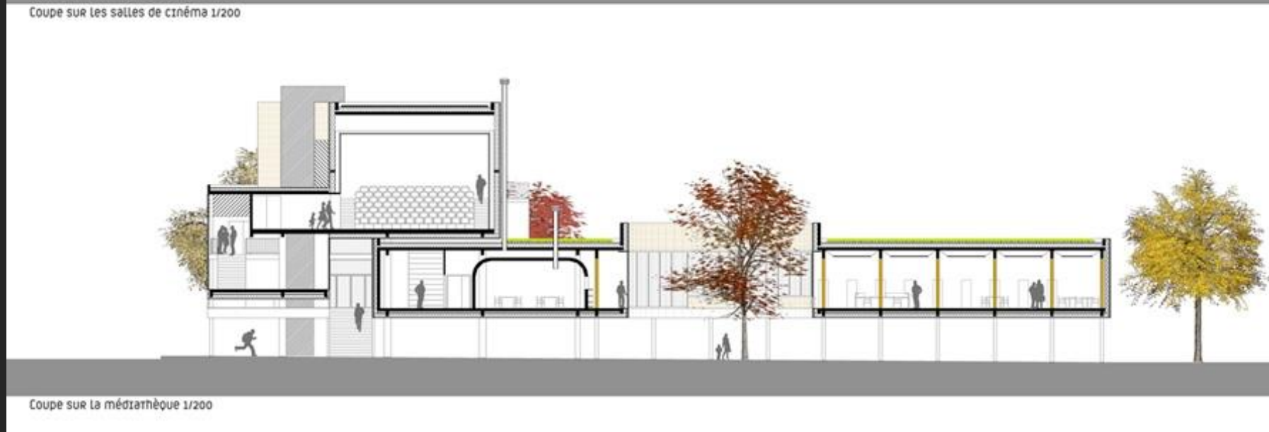
Coupe sur les salles de cinéma 1/200
